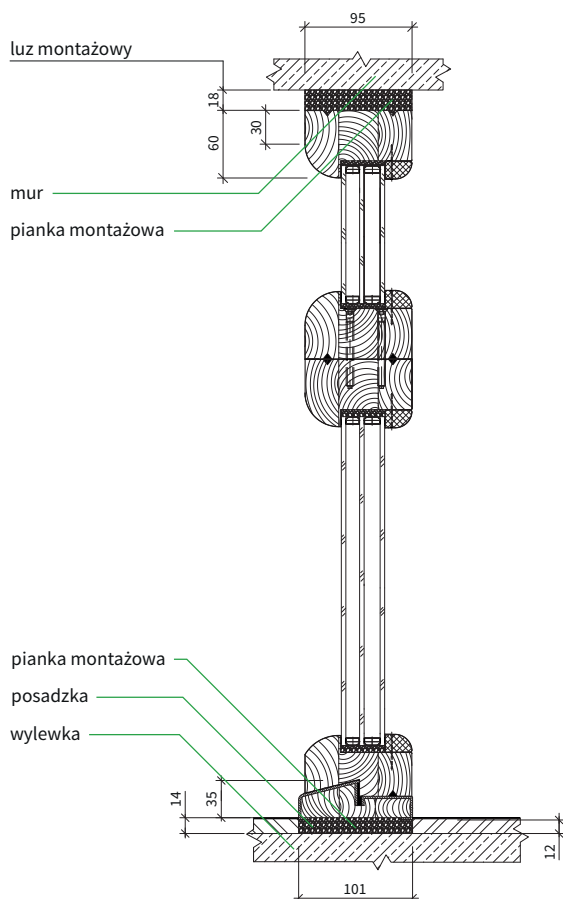
Przekrój przez dostawkę boczną
