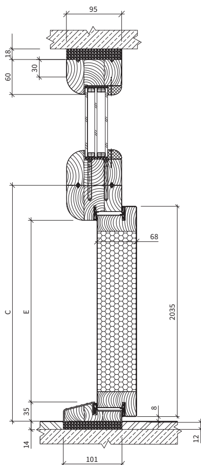
Przekrój przez skrzydło
